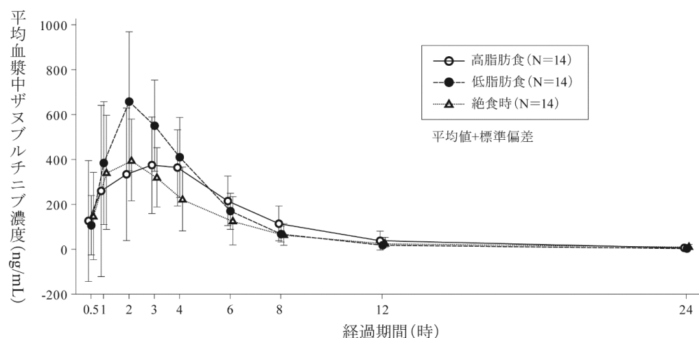
食事の状態別の血漿中ザヌブルチニブ濃度推移
