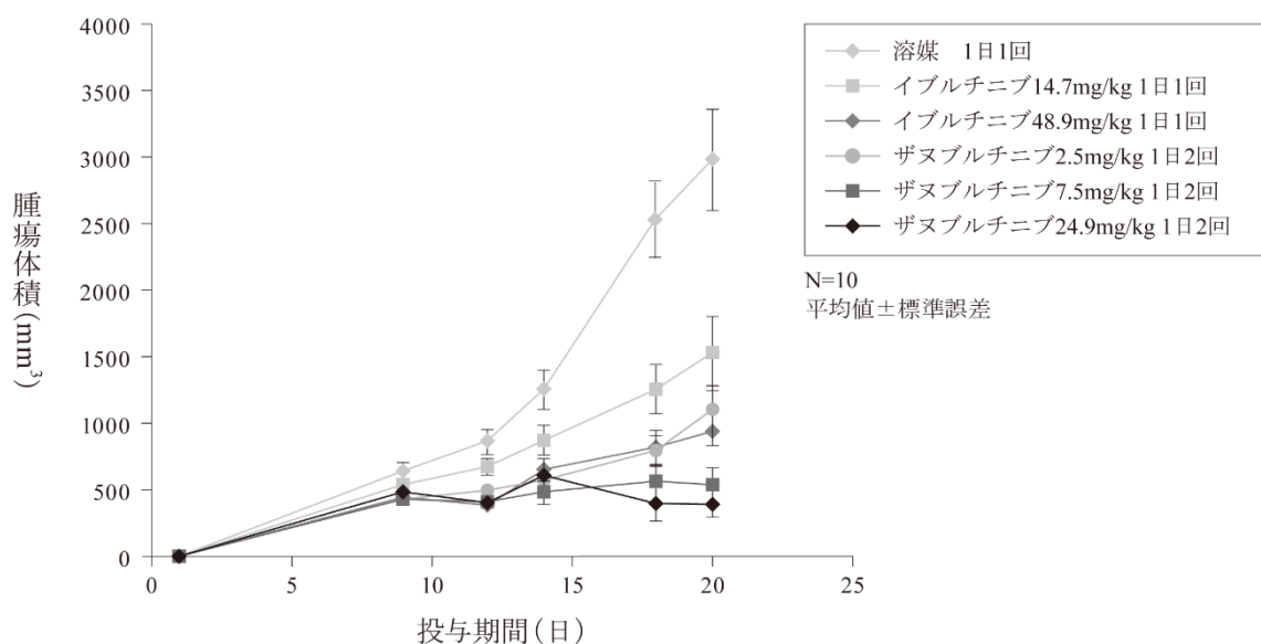
ザヌブルチニブ用量別の腫瘍体積の推移
