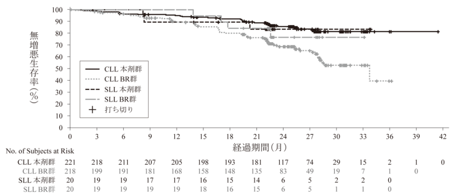
コホート 1 における病型別 PFS（IRC 判定）
